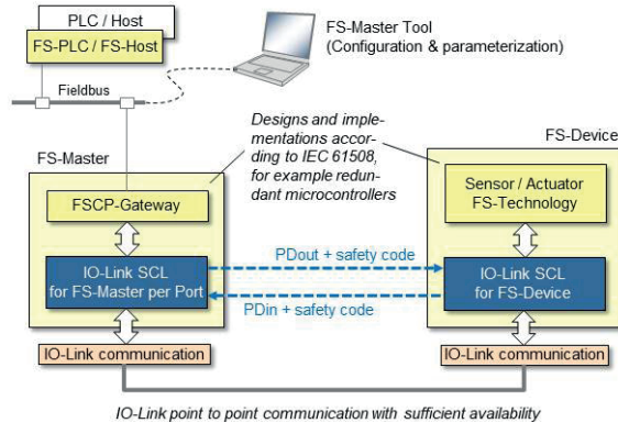
Fig. 8: SCL layer stacks
